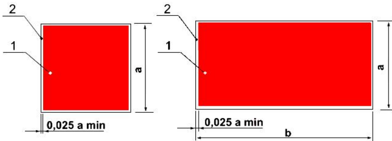
Рисунок 4. Основа цветографического изображения и соотношение размеров знаков пожарной безопасности
